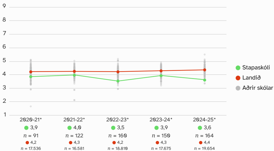
2.1. Sjálfsálit — Ársmeðaltöl
